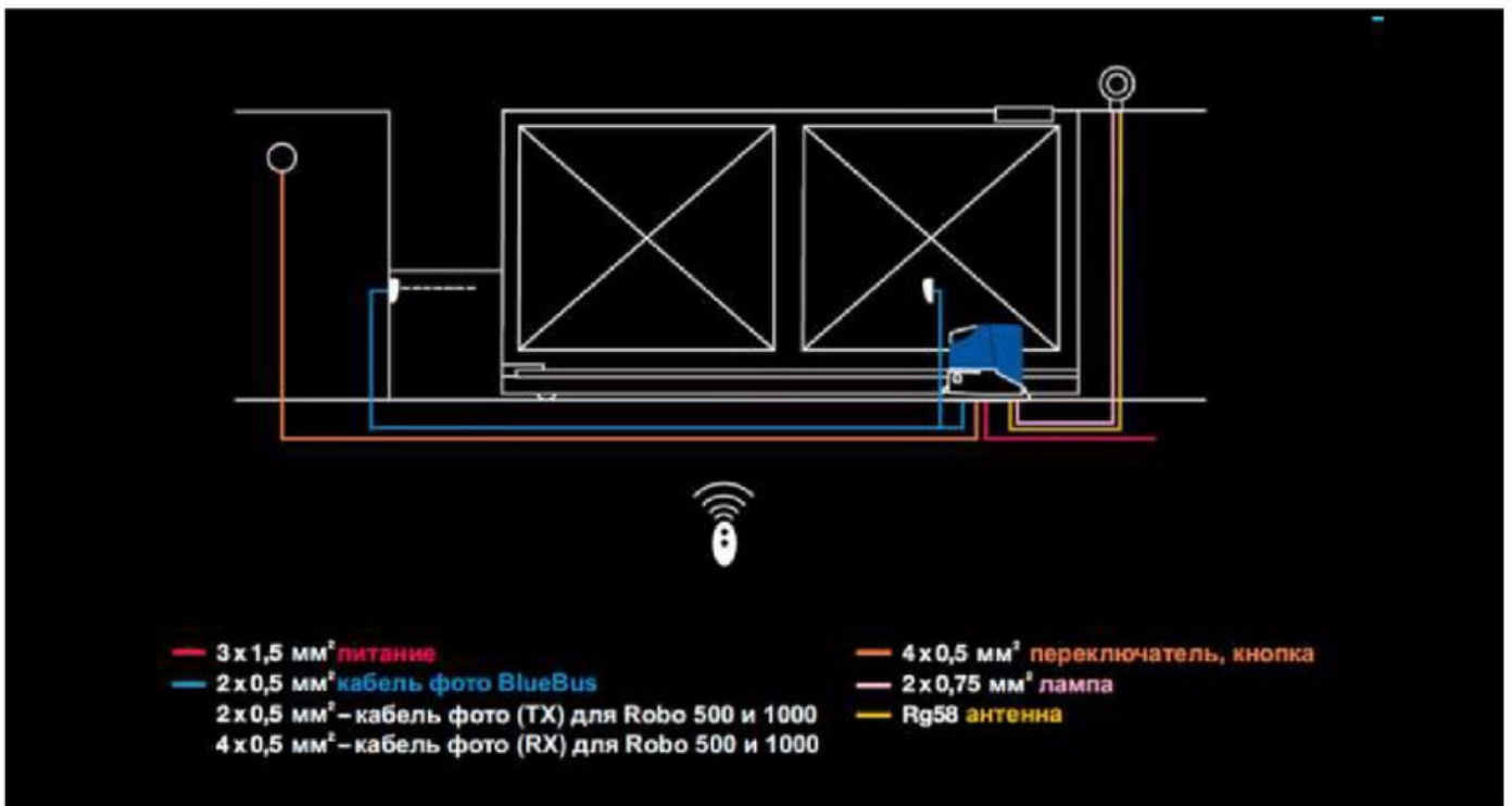
Схема проводки питания
